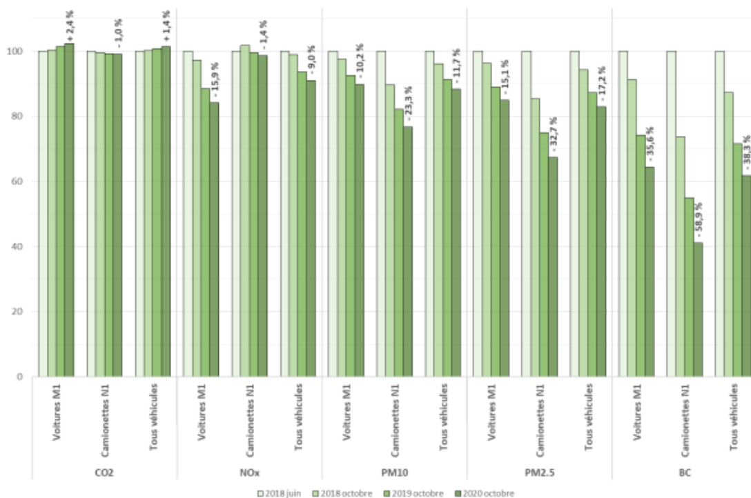
Gràfic 12 Evolució de les emissions del transport per carretera a partir de dades de càmeres entre juny de 2018 i octubre de 2020 en un escenari amb quilòmetres recorreguts constants a Brussel·les [51]
